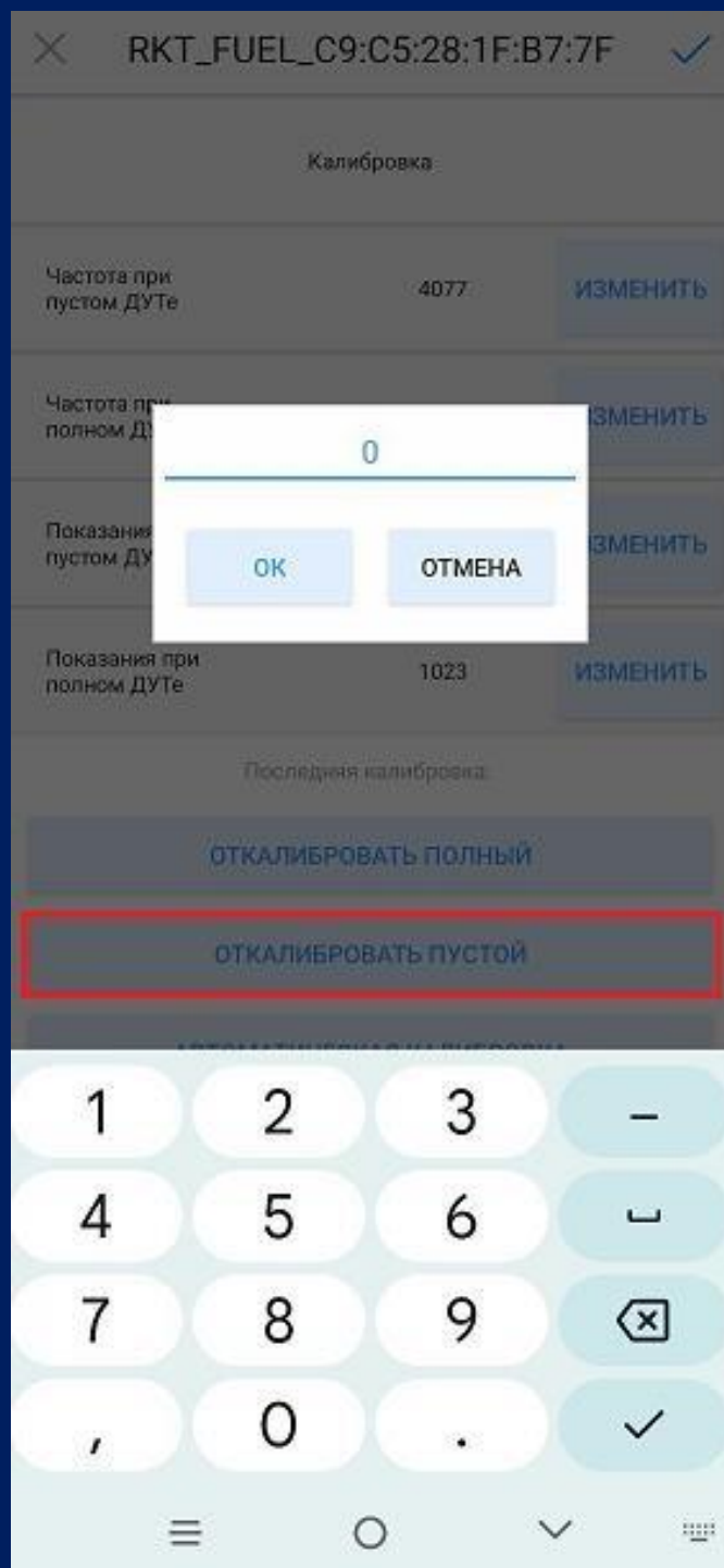
Рисунок 11 – Калибровка пустого
