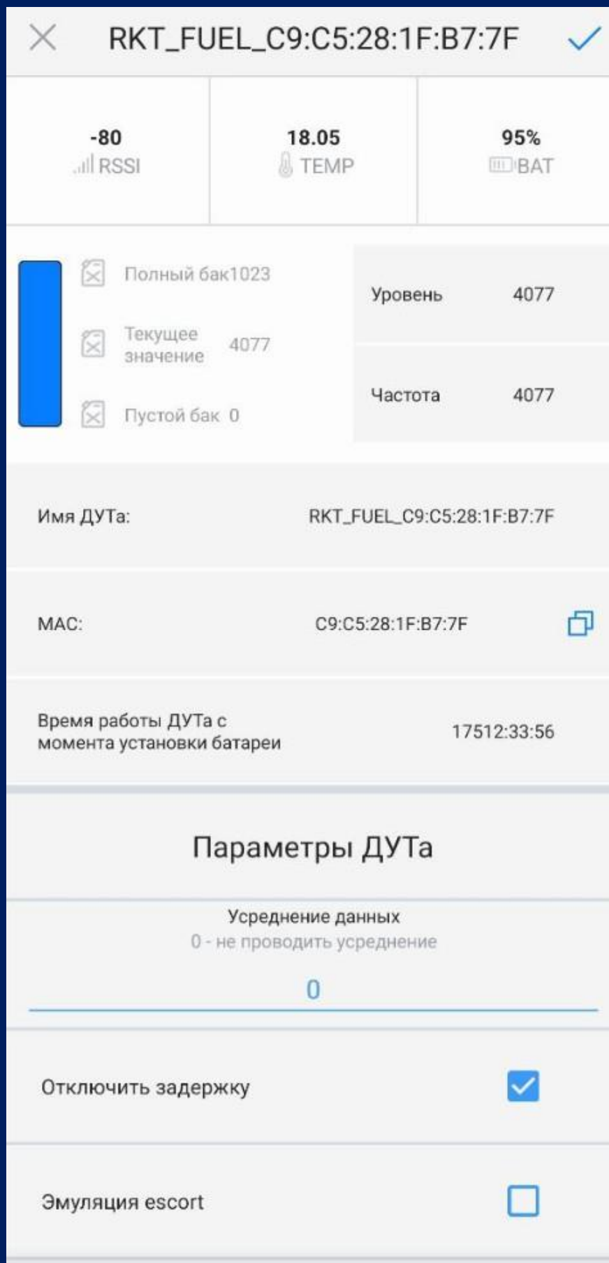
Рисунок 9 – Окно настройки ДУТ BLE
