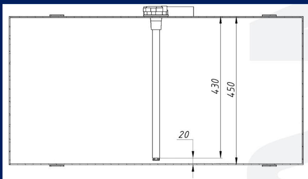
Рисунок 5 – Обрезанный ДУТ ВЛЕ, смонтированный на топливный бак
